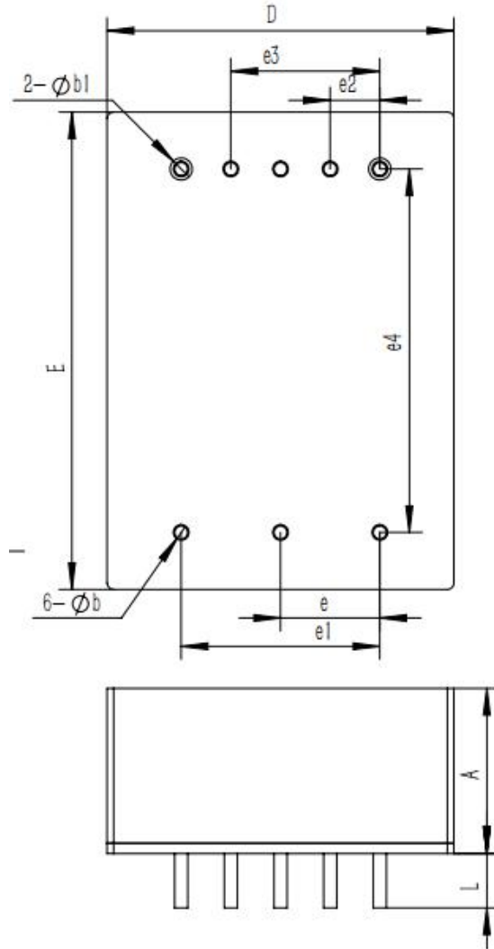
传统五面金属体封装外形尺寸
