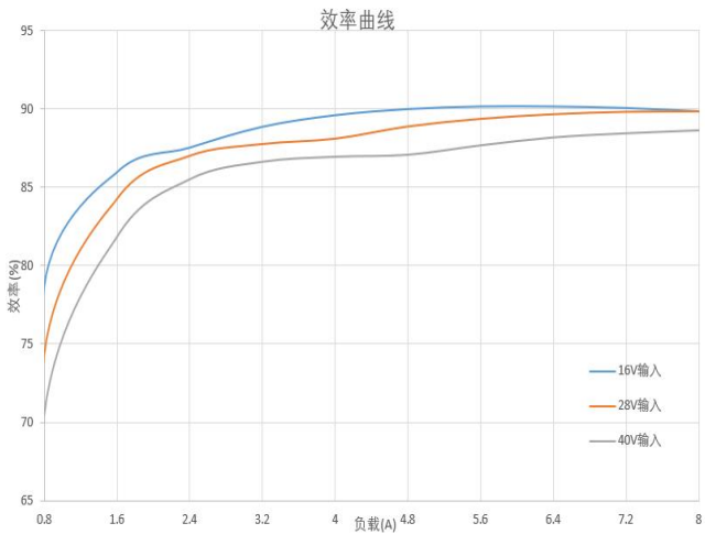
图1 效率曲线
