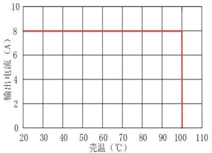
图 6 降额曲线
