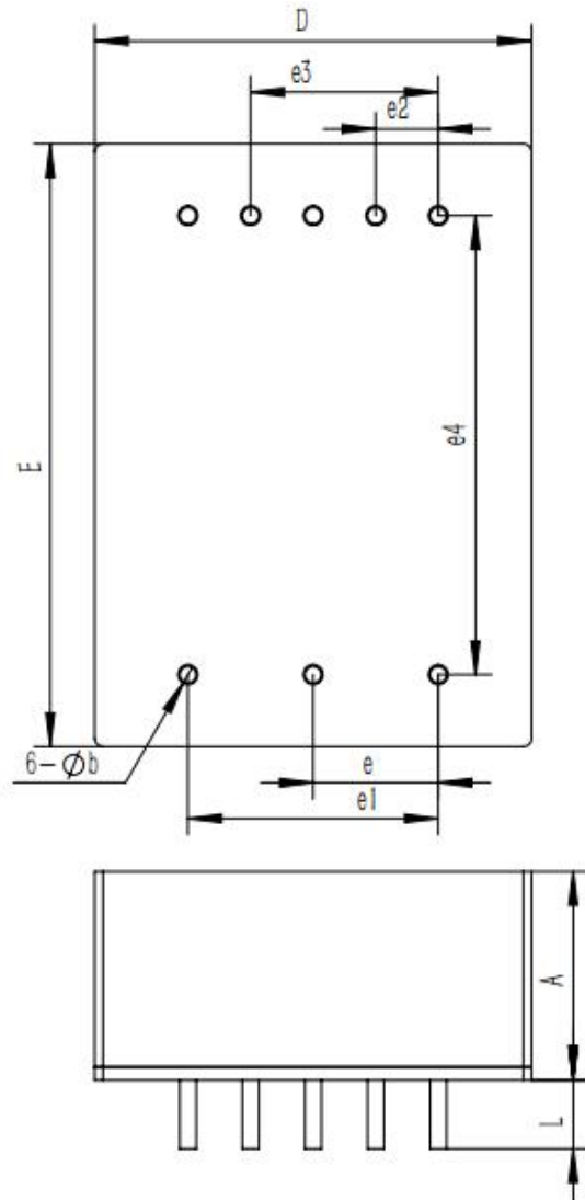
外形尺寸
