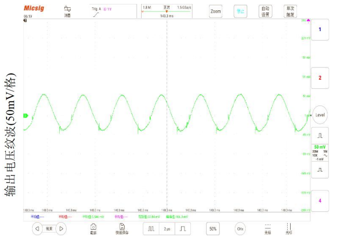
图4 输出电压纹波
