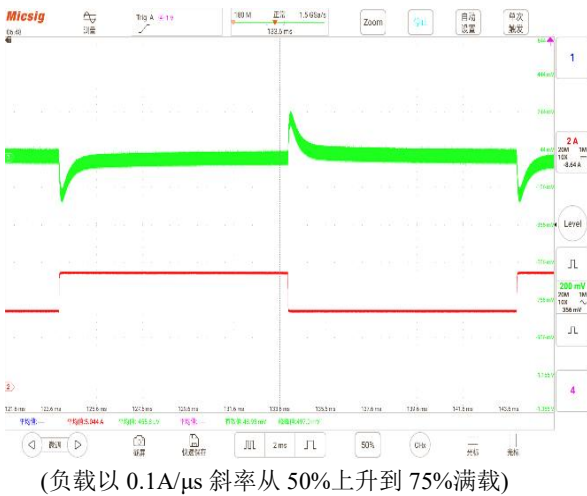
图 5 动态响应
