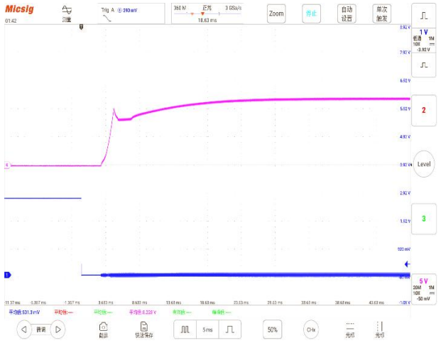
图3 使能控制开启响应
