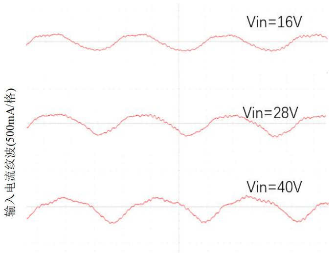
时间 (1μs/格)
